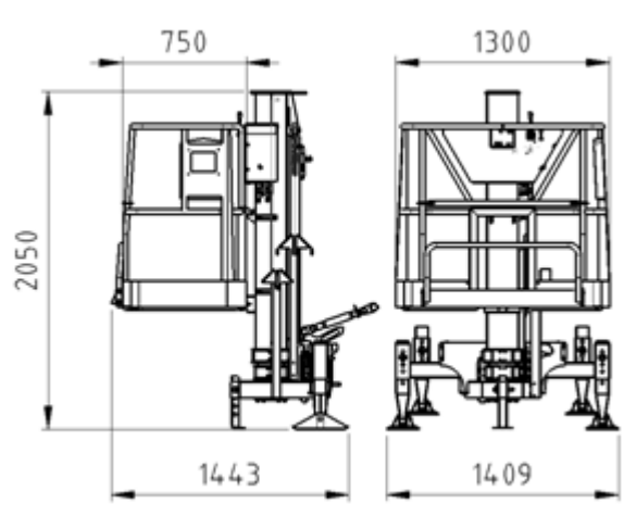
Rysunek 1 – Platforma robocza Leguan 50 w pozycji transportowej
