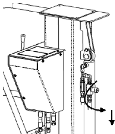
Zawór opuszczania awaryjnego na platformie
